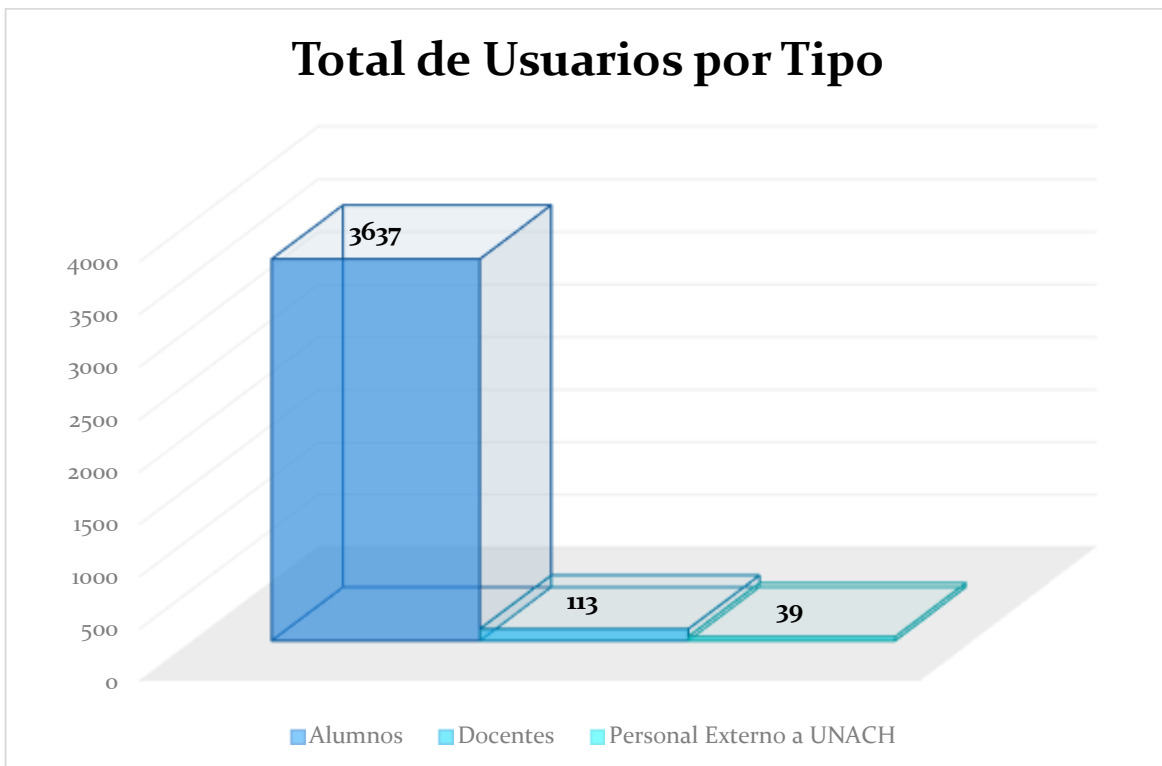
Graf. 2 Total de Alumnos, Docentes, Personas Externas a la UNACH
