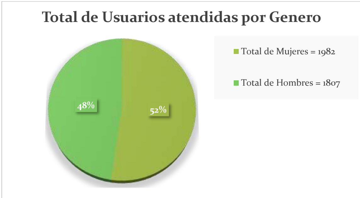
Graf. 1 Total de Usuarios por Género
