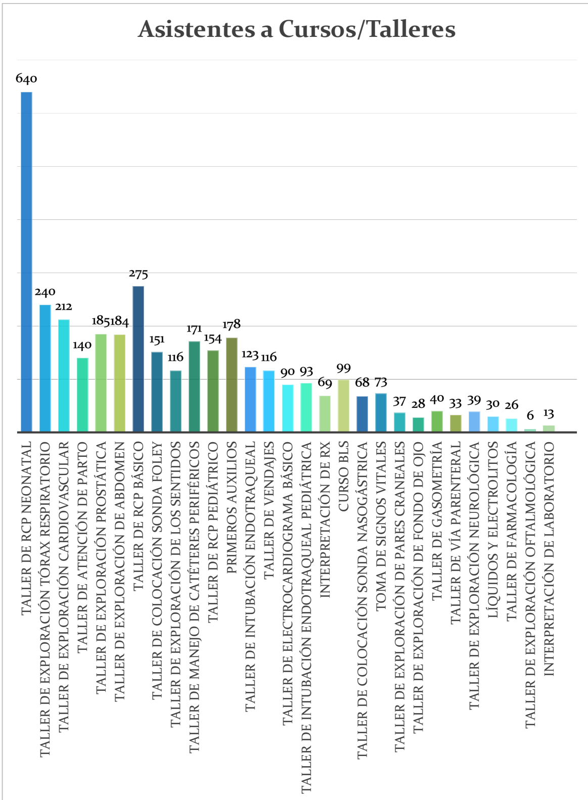
Graf.7 Aforo por Taller/Curso/Clase Impartida
