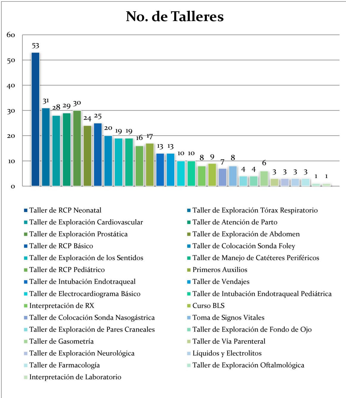
Graf. 8 Total de Talleres impartidos
