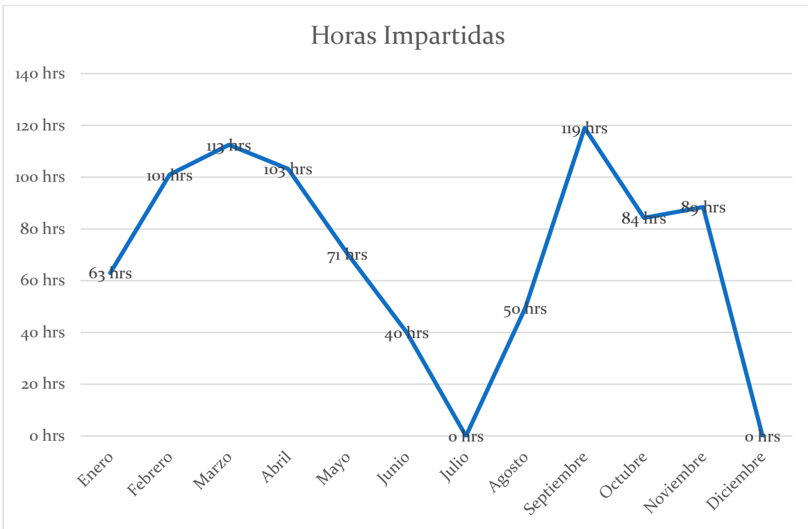
Graf. 4 Total de horas impartidas en la UCAM
