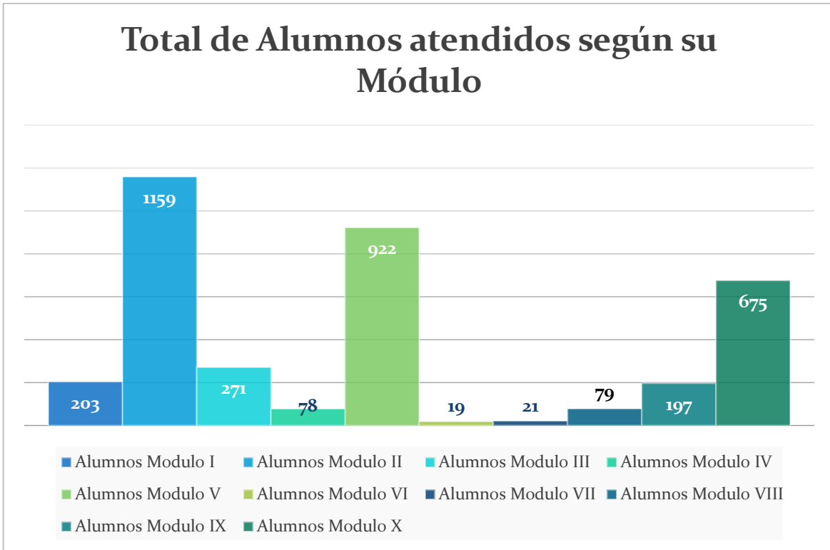
Graf. 5 Total de Alumnos por Modulo
