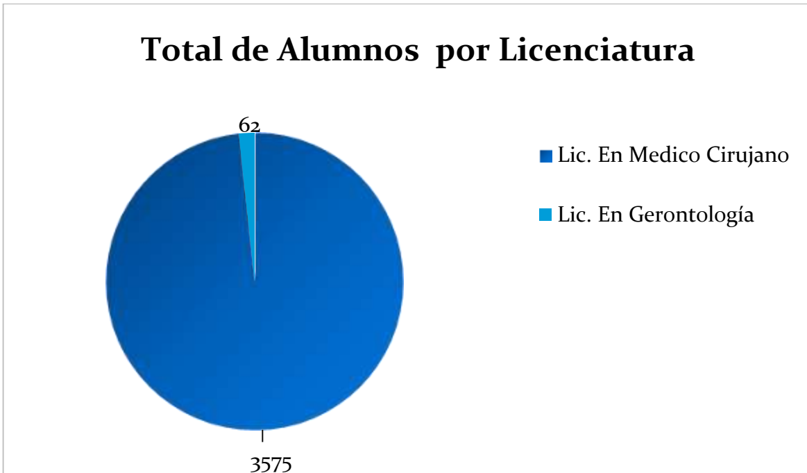
Graf. 6. Total de alumnos por Licenciatura.
