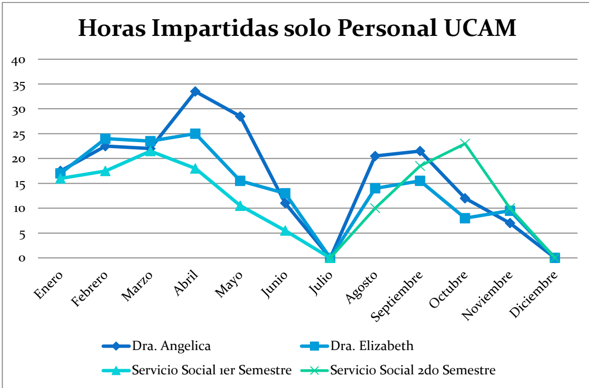
Graf. 8 Distribución total de horas impartidas por personal adscrito a UCAM
