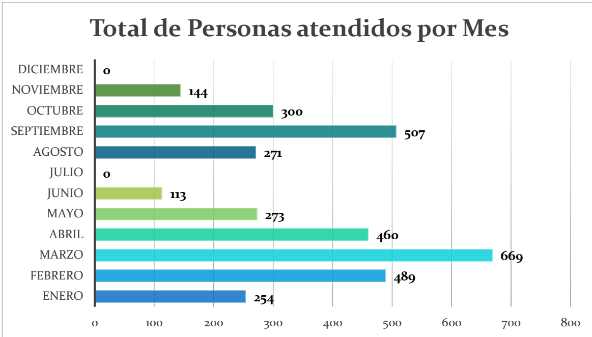
Graf. 3 Total de Aforo por Mes
